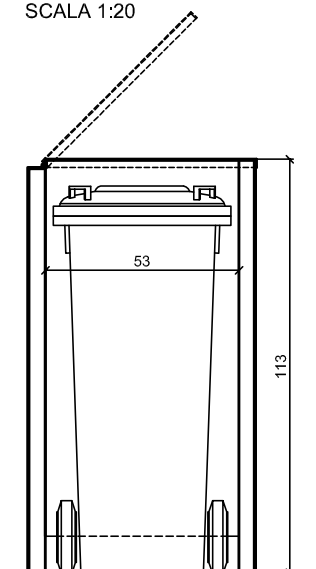
SEZIONE VERTICALE SCALA 1:20
