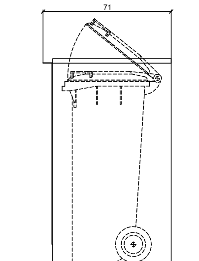
PROSPETTO LATERALE SCALA 1:20
